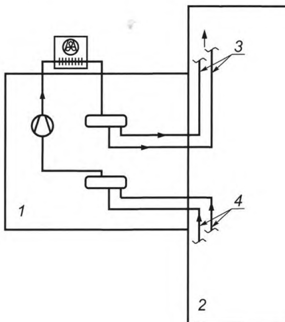
Рисунок С.2 — Холодильная система со всеми элементами, содержащими хладагент, установлена в машинном отделении или на открытом воздухе
