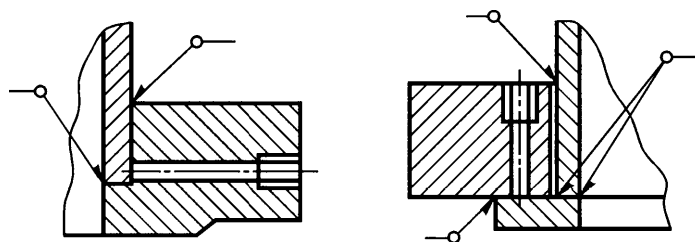
а — для исполнений 1—5; б — для исполнений 6—10
