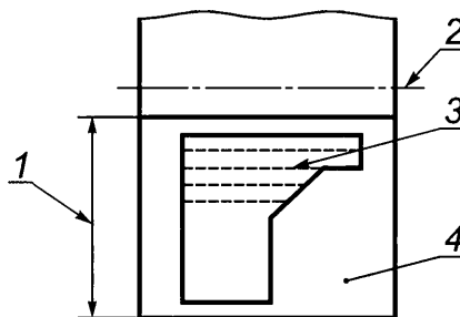
1 — толщина заготовки; 2 — ось фланца; 3 — волокно; 4 — лист или сортовой прокат
