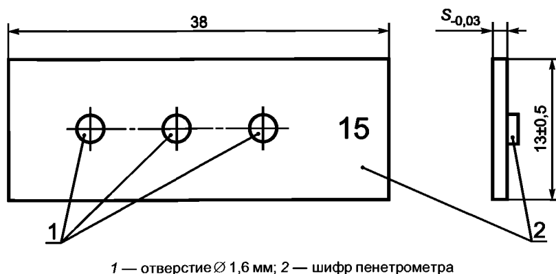
Рисунок Б.1 — Стандартный пластинчатый пенетрометр
