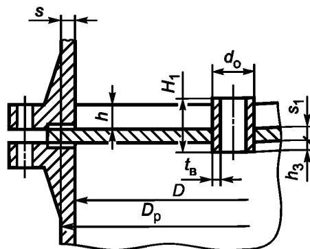
Рисунок 24 — Плоская круглая пластина с радиальными ребрами жесткости
