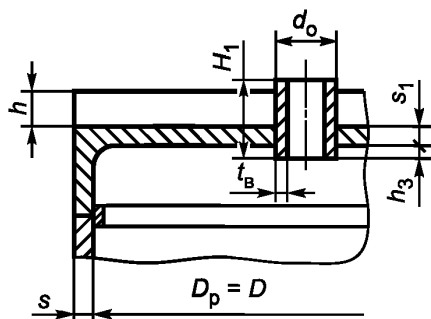
Рисунок 23 — Плоское круглое днище с радиальными ребрами жесткости
