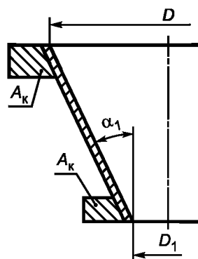
Рисунок 29 — Коническая обечайка с кольцами жесткости
