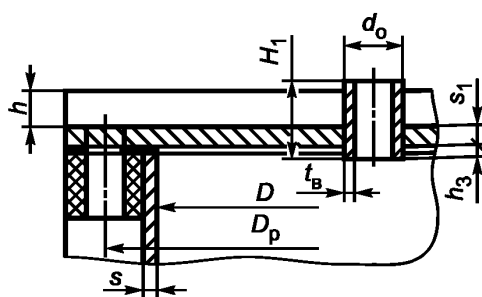
Рисунок 22 — Плоская круглая крышка с радиальными ребрами жесткости
