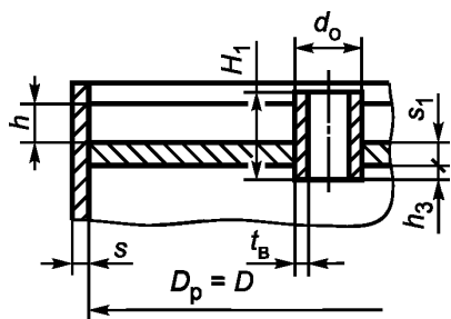
Рисунок 21 — Плоское круглое днище с радиальными ребрами жесткости
